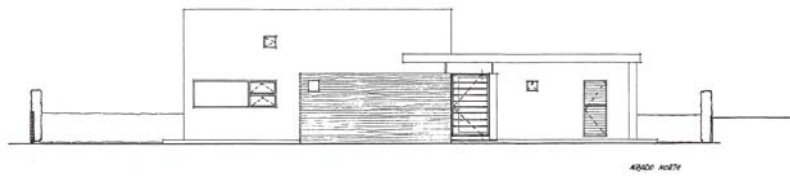
Alzados N y S
