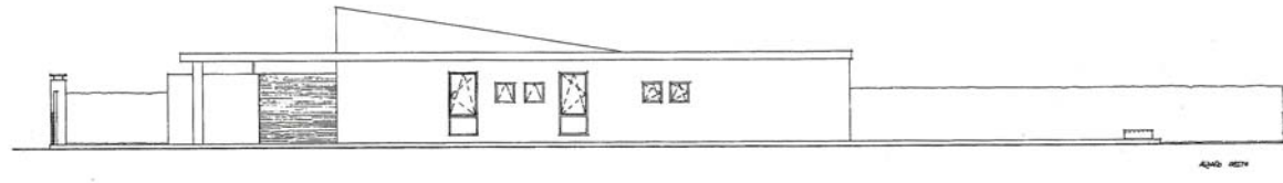
Alzados E y W
